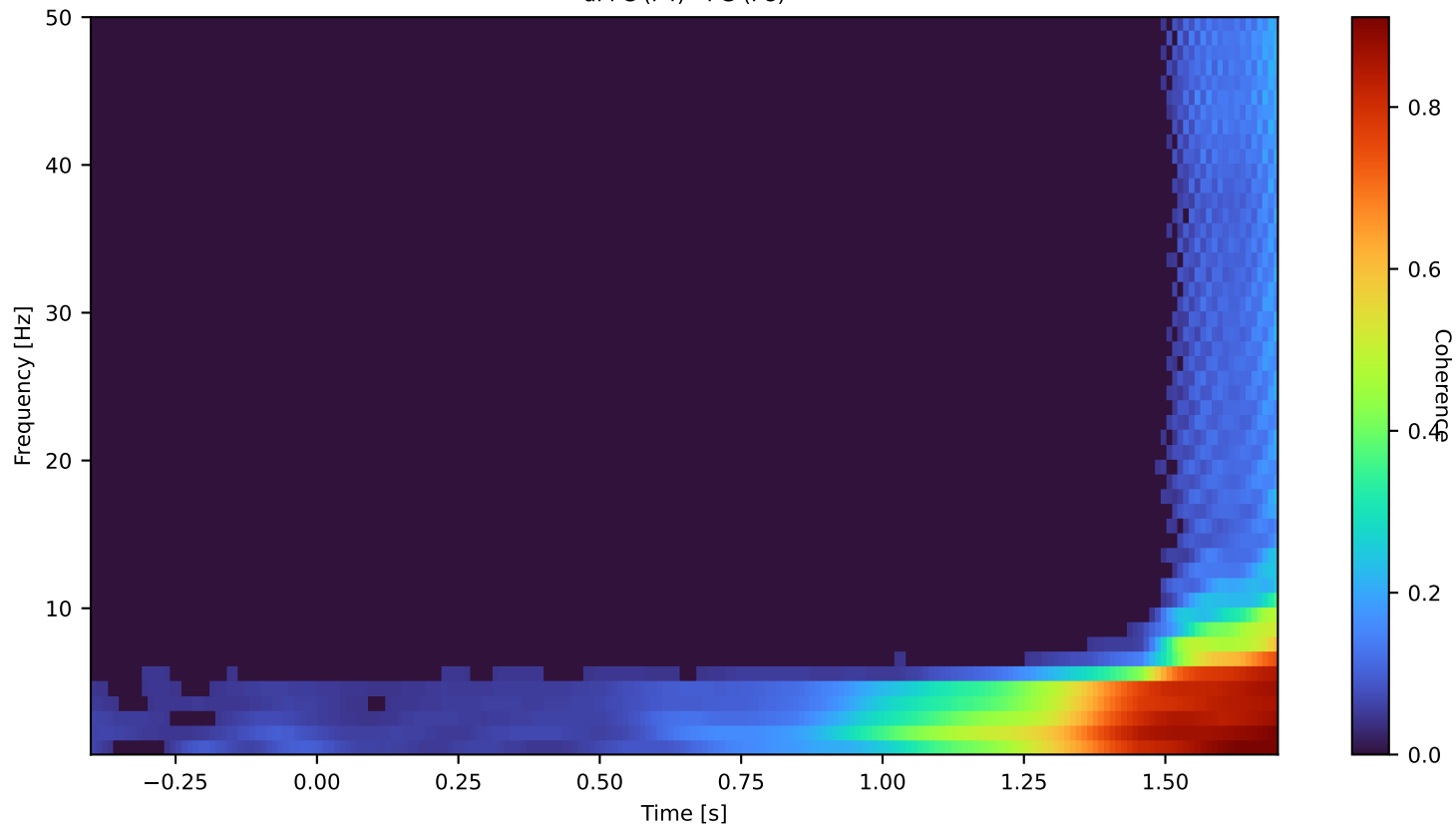
dPFC (F4) - PG (P8)
